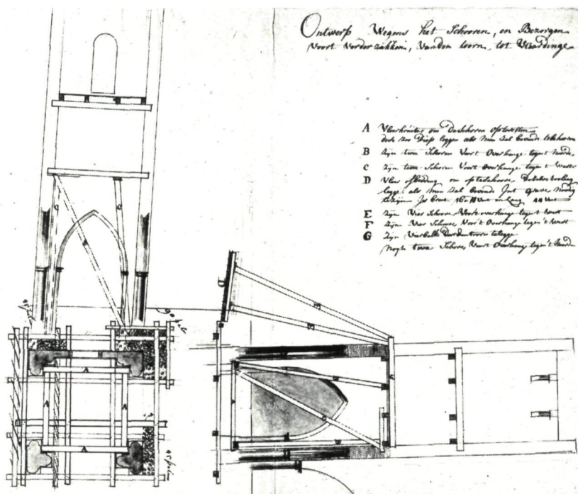
Plan van David van Stolk om verder scheef zakken van de toren van Vlaardingen te voorkomen, 1734
