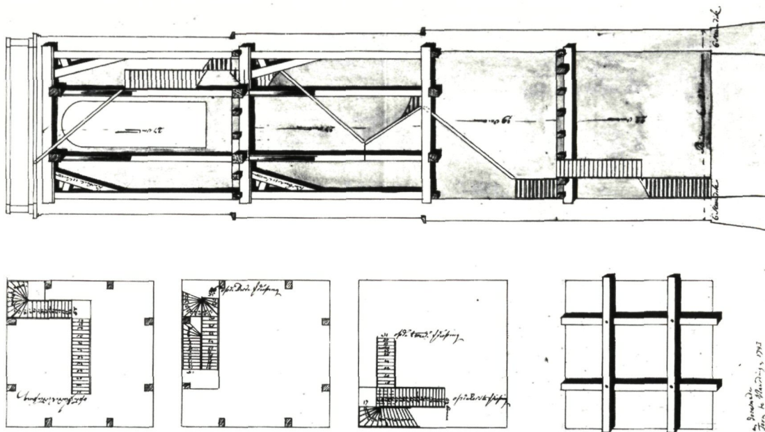
Plan van David van Stolk om verder scheef zakken van de toren van Vlaardingen te voorkomen, 1734
