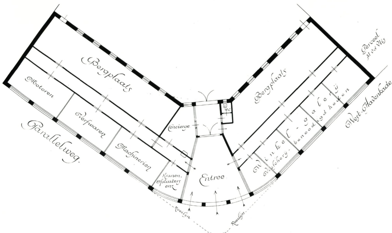
Plattegrond en opstandtekening van een “Fabriek van geoliede goederen en visscherijbenoodigheden” aan de Parallelweg, hoek Westhavenkade, door A. Maarleveld voor Jacob van Toor. Opvallend is de halfronde entree op de hoek, die in de opstandtekening is terug te vinden onder de vlaggen. 1912.
