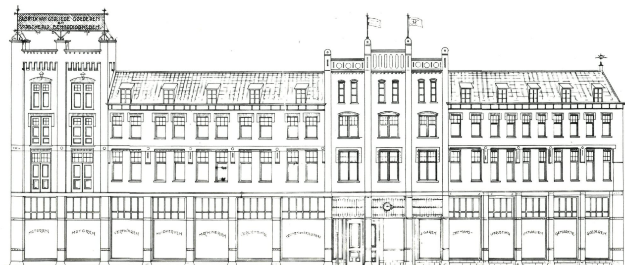
Plattegrond en opstandtekening van een “Fabriek van geoliede goederen en visscherijbenoodigheden” aan de Parallelweg, hoek Westhavenkade, door A. Maarleveld voor Jacob van Toor. Opvallend is de halfronde entree op de hoek, die in de opstandtekening is terug te vinden onder de vlaggen. 1912.
