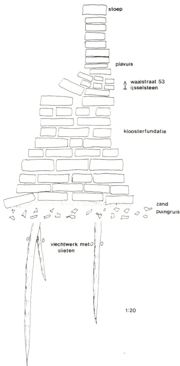
Doorsnede door het fundament van een van de kloostermuren (waarschijnlijk zuster- of weeshuis), waarop in de late 16e eeuw een klein woonhuis werd gebouwd (Waalstraat 53)
