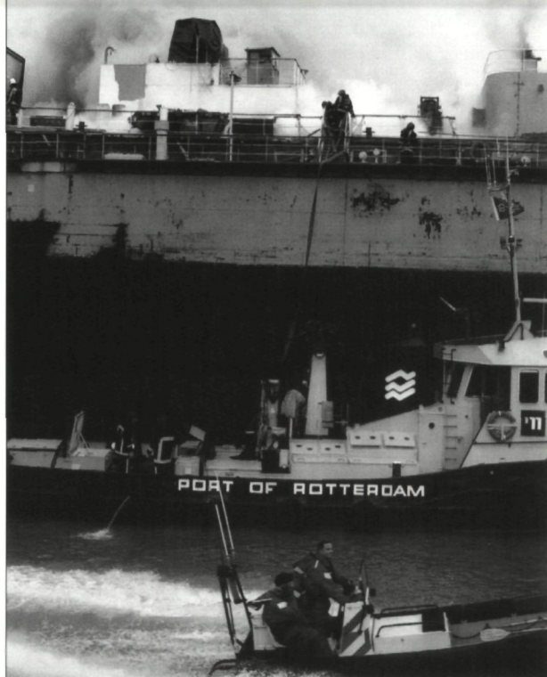
Groot alarm na een scheepsbrand in de Vulcaanhaven (6 maart). (Foto Roel Dijkstra).
