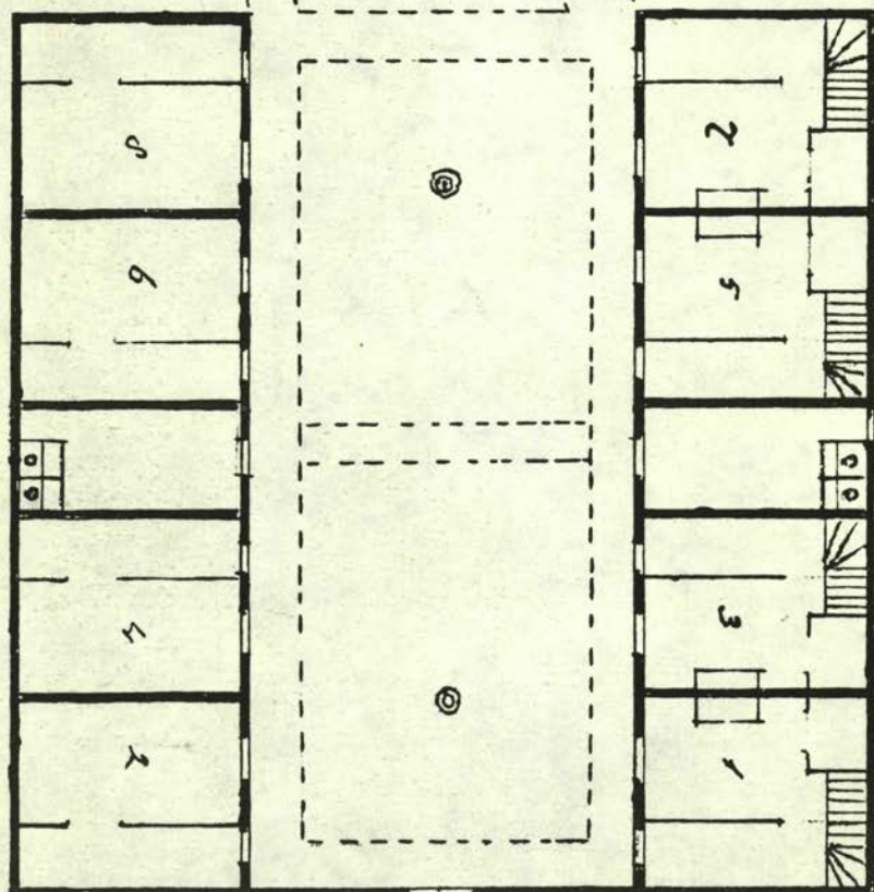
Plattegrond van het Van Leydenshofje ca 1900. Schaal 1:200. Onderaan de ingang aan het Veerplein. Inv. van het archief Van Leydenshofje nr 41.
