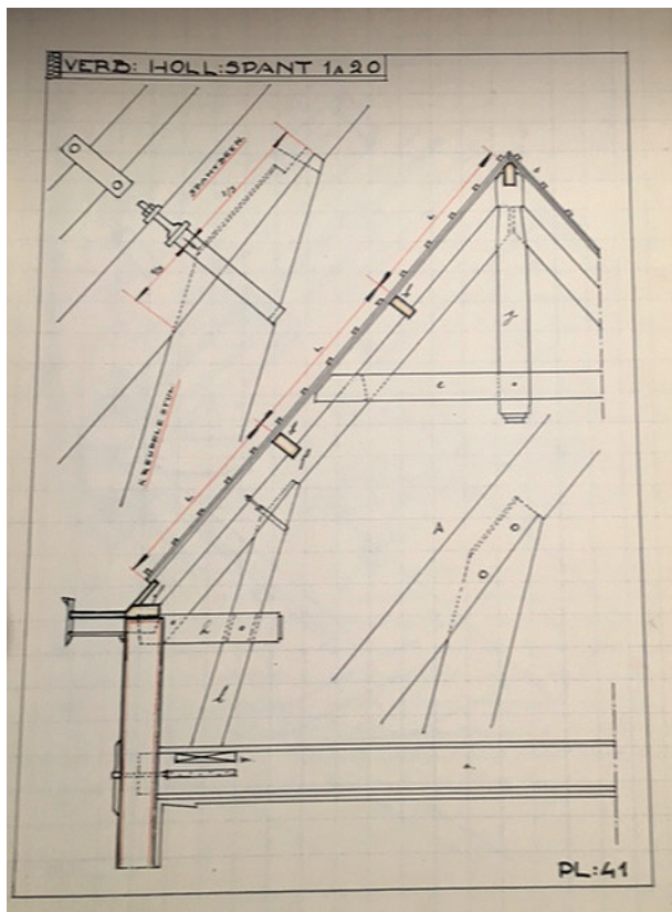
Tekening van A. den Hoedt die in het cursusjaar 1935/36 het vak timmeren volgde op de Vlaardingse Ambachtsschool. Collectie A. den Hoedt.
